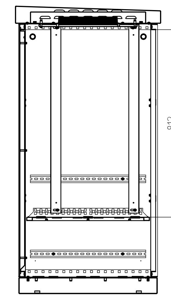
ШТВ-1-18U.6.6-4AAA
