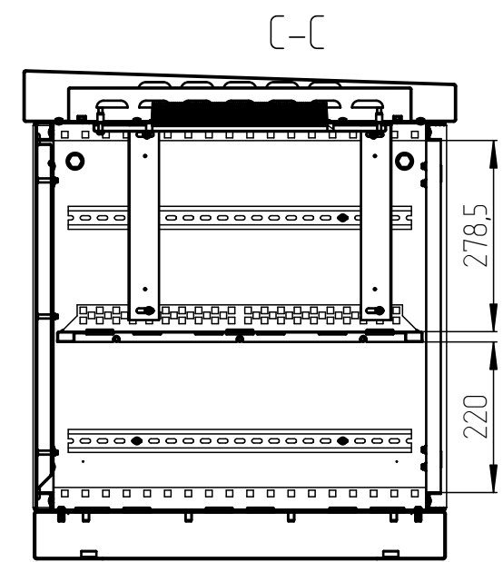
ШТВ-1-6U.6.6-4AAA
