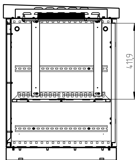
ШТВ-1-12U.6.6-4AAA
