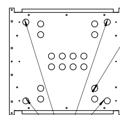
Основание каркаса ШТВ-1-х6.6
