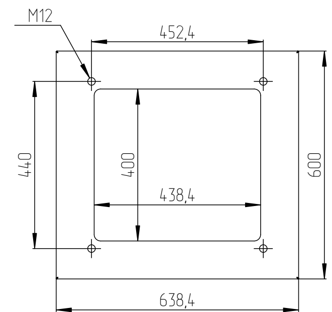
Основание шкафа ШТВ-1-х6.6
