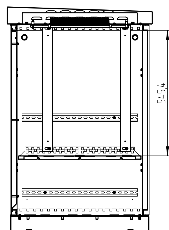
ШТВ-1-15U.6.6-4AAA
