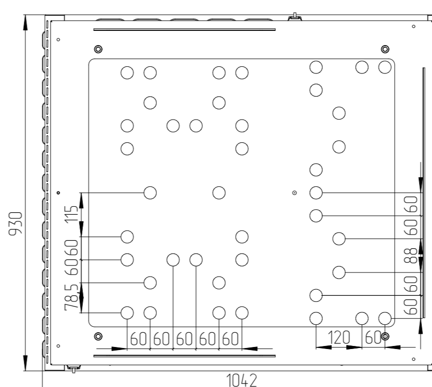
Вид снизу и габариты по крыше
